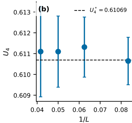
Binder cumulant
