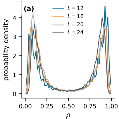
Critical P_L(\rho)
